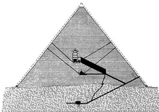
Nákres řezu vnitřku Velké pyramidy.
